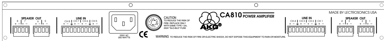
Abbildung 7 - CA810 Rückwand
